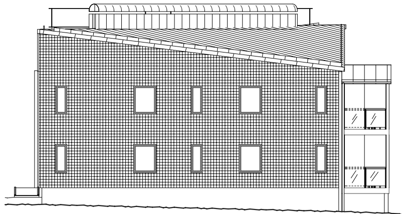
FASAD HUS A2 MOT NORR
