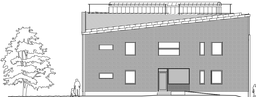
FASAD HUS A2 MOT ÖSTER
