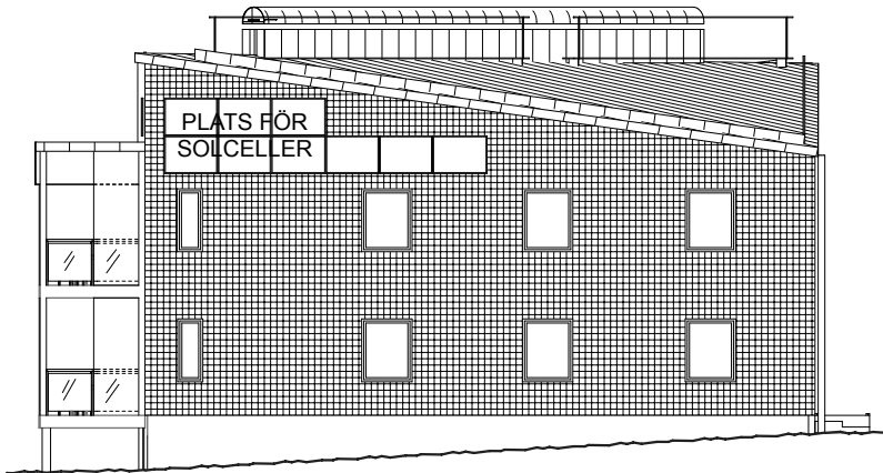
FASAD HUS A2 MOT SÖDER
